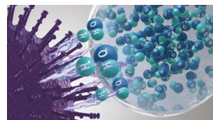
Hydroxylradikaler denaturerer proteinerne i forurenende stoffer.
